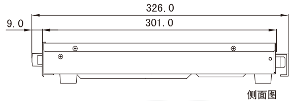
侧面图
